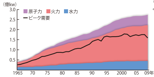
「電力のピーク需要」と「発電能力」
